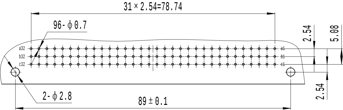
插头安装孔尺寸
