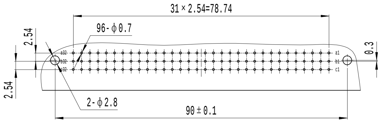
插座安装孔尺寸
