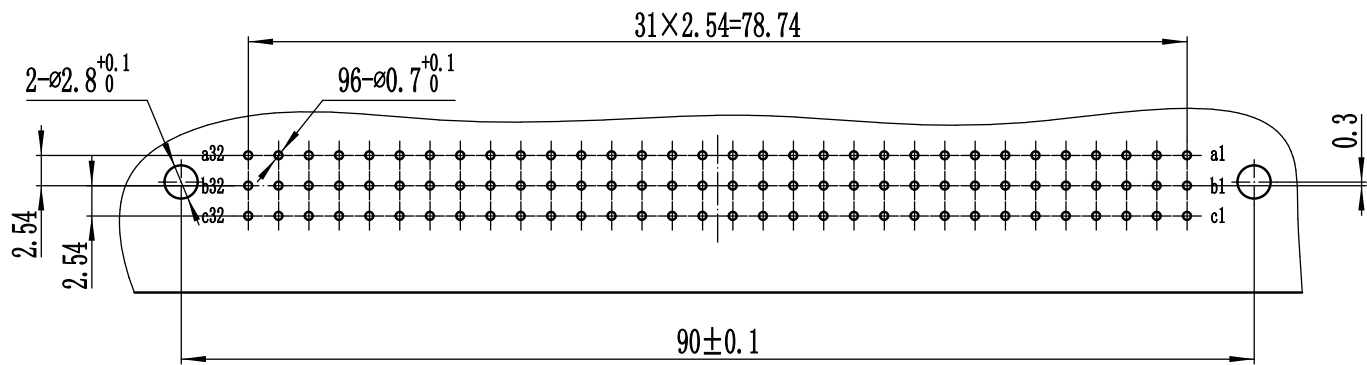
插座安装孔尺寸
