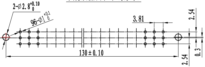
印制板安装开孔尺寸 (供参考)
