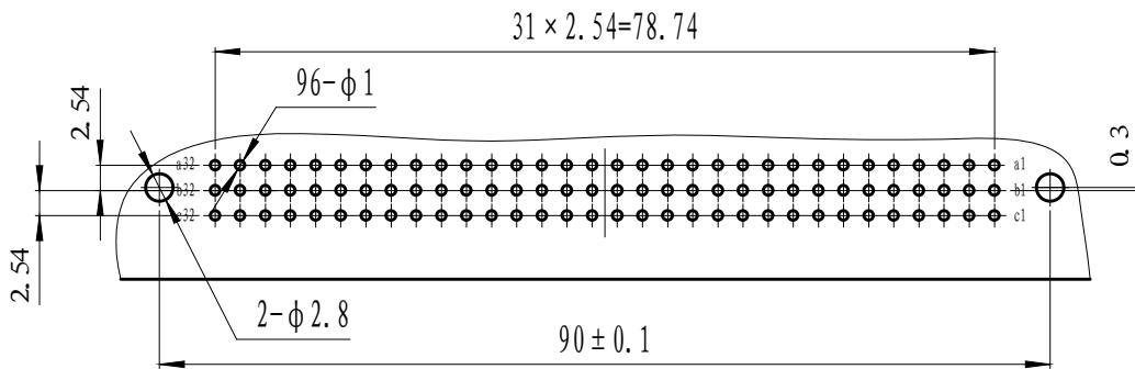
插座安装孔尺寸
